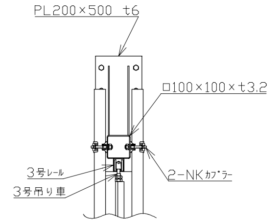
A部詳細 (1/16)
