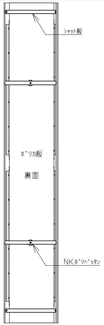
ホリカ板取付イメージ図 1/20
