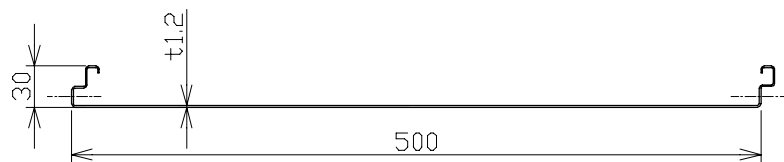
A矢視図 1/5
