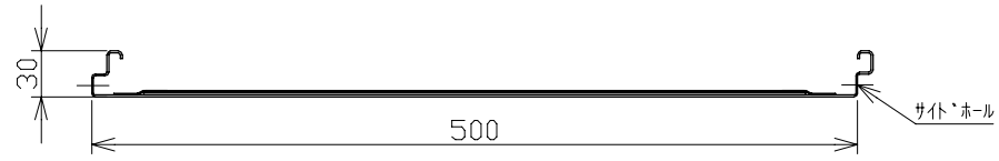
A矢视图 1/5
