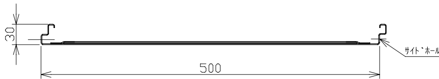
A矢视图 1/5
