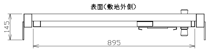
A矢视图 1/10
