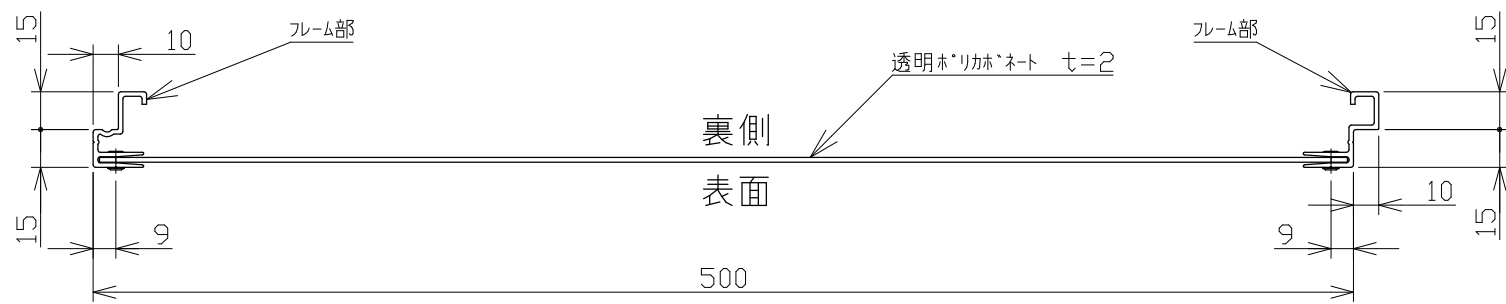
A矢視図 (1/3)
