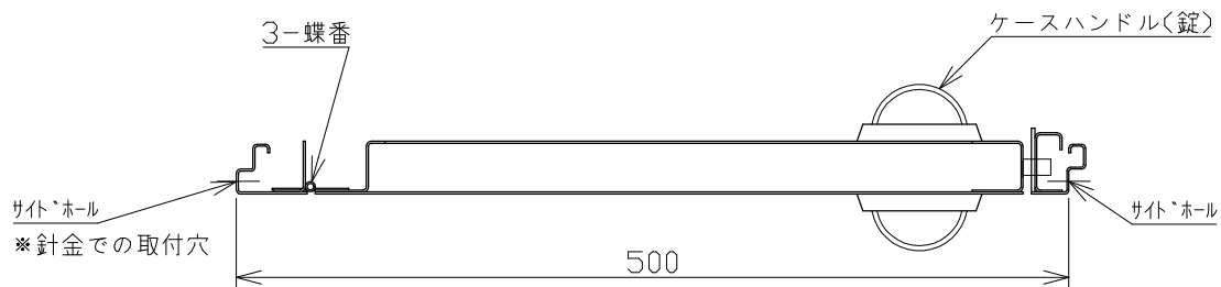
A矢视图 1/5
