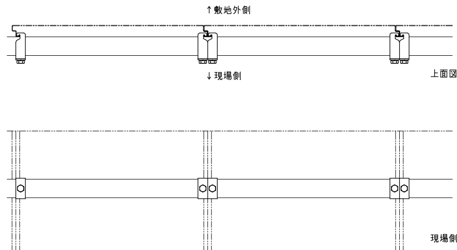
組付時参考図 1/10
