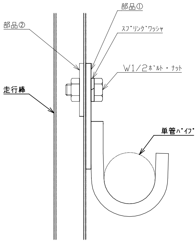
取付けイメージ図 1/2
