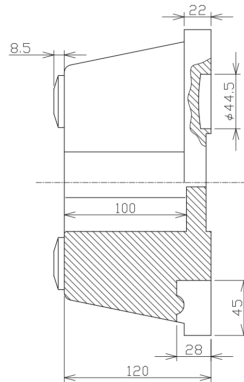
A-A'断面・矢視図
