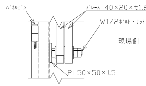
B部詳細 1/5
