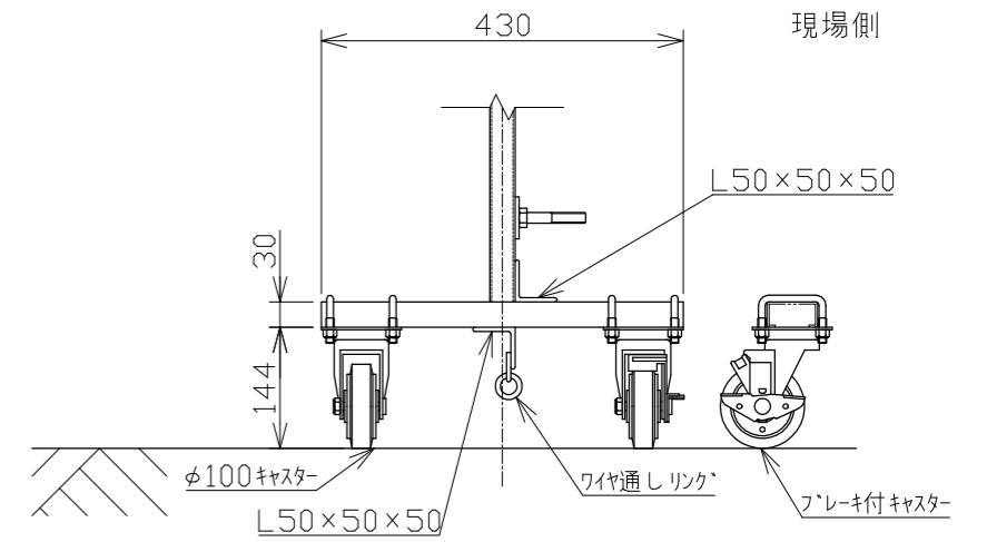
軸足(フレイキ付き) 1/10
