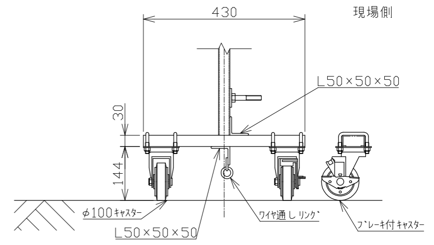
軸足(フレキ付き) 1/10
