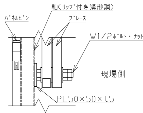
B矢視図 1/5
