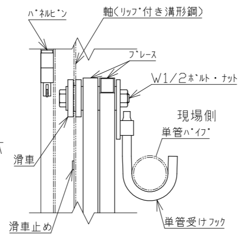
A矢視図 1/5
