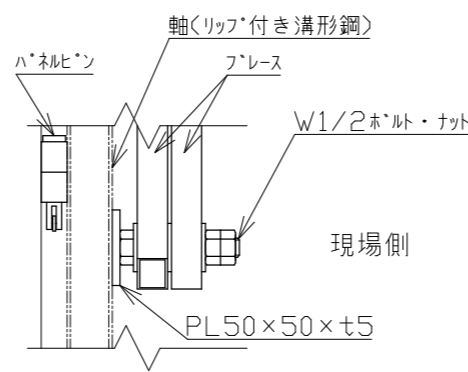
B矢視図 1/5
