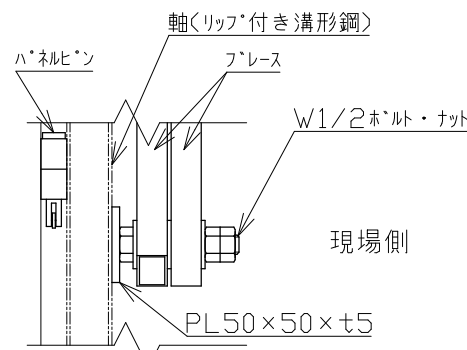
A矢視図 1/5
