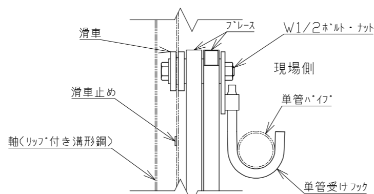
A矢視図 1/5
