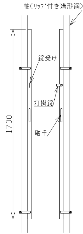
施錠用金具 (オプション) 1/20
