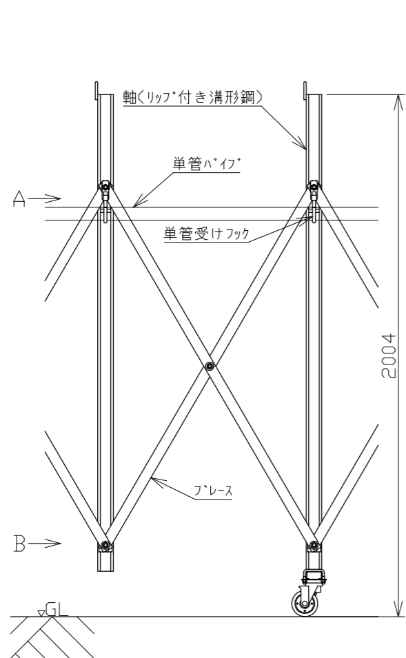
背面図<フレス> 1/20
