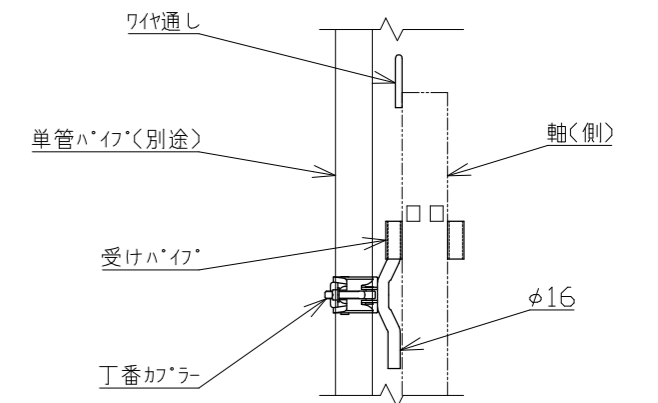
丁番カチラー部分詳細 1/10
