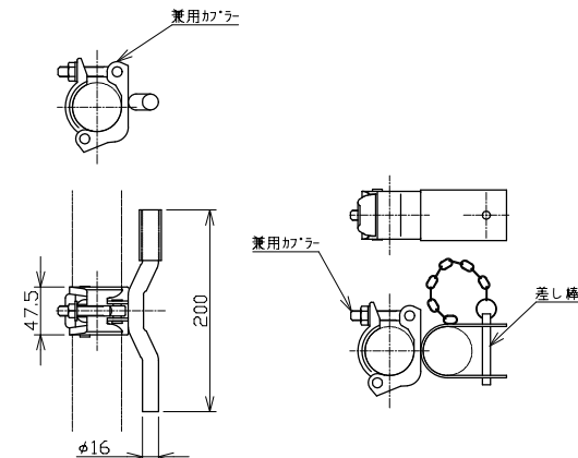
A部詳細 1/5 丁番カフラー B部詳細 1/5 ロックカフラー ※オプション
