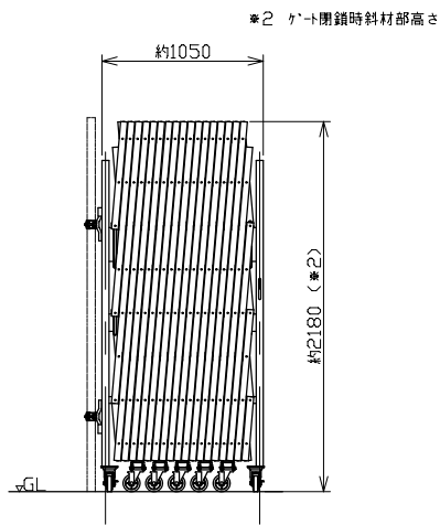
ケート解放時 1/30
