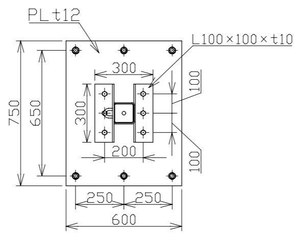
C-C'矢視図 1/20
