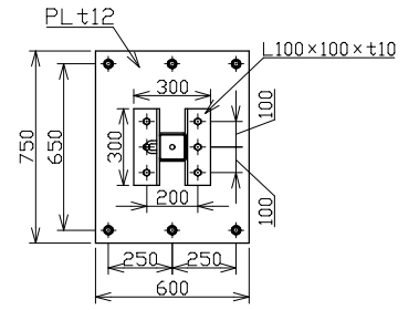
C-C'矢视图 1/20
