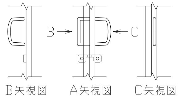
取手部分詳細 1/10
