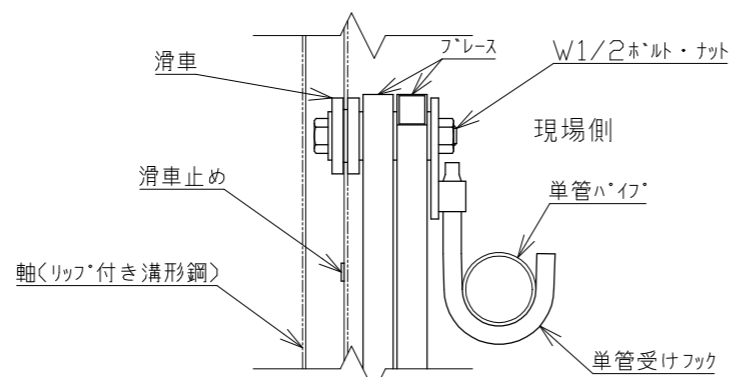
A矢視図 1/5
