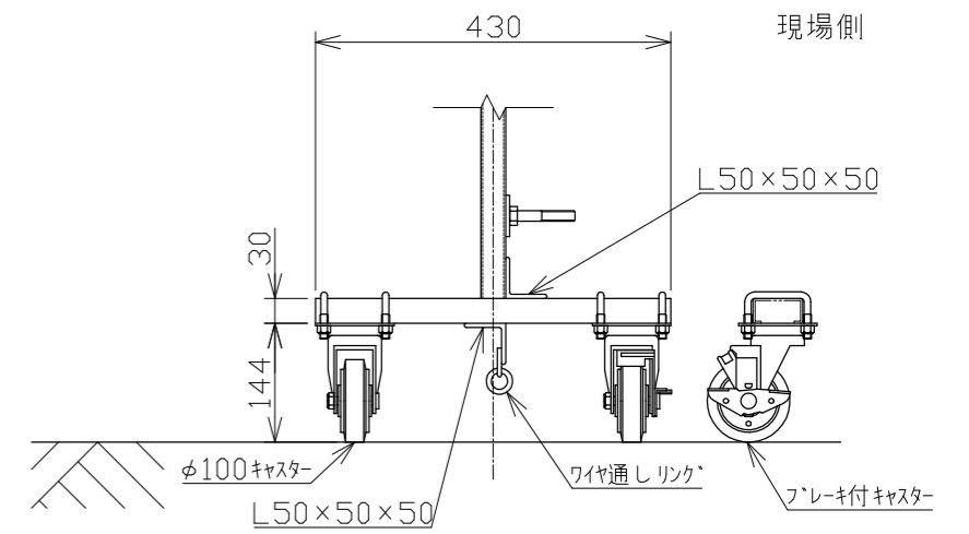
軸足(ブレーキ付き) 1/10
