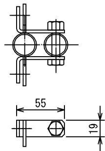
掛け金部 詳細
