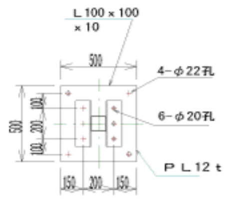
矢視 A-A 1/20
