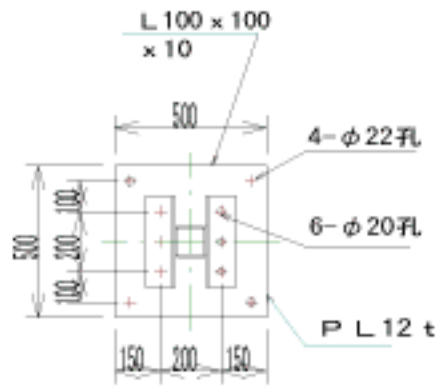
矢視 A-A 1/20
