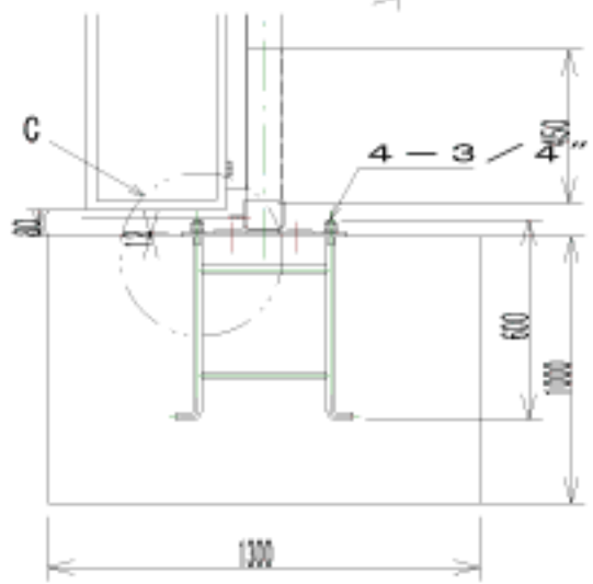
詳細 D 1/20
