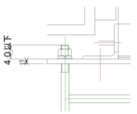
詳細 C 1/5
