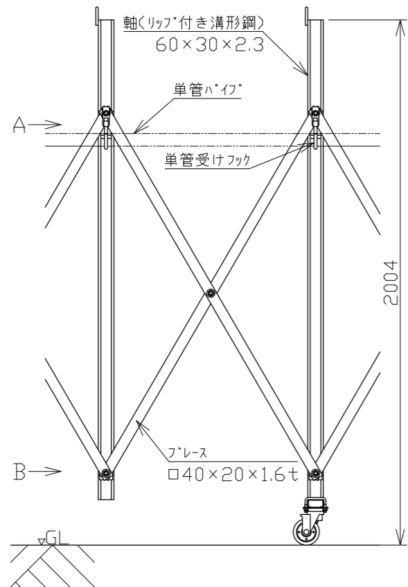
背面図(プレス) 1/20
