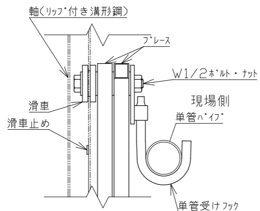
A矢視図 1/5
