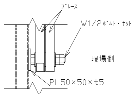
B矢視図 1/5
