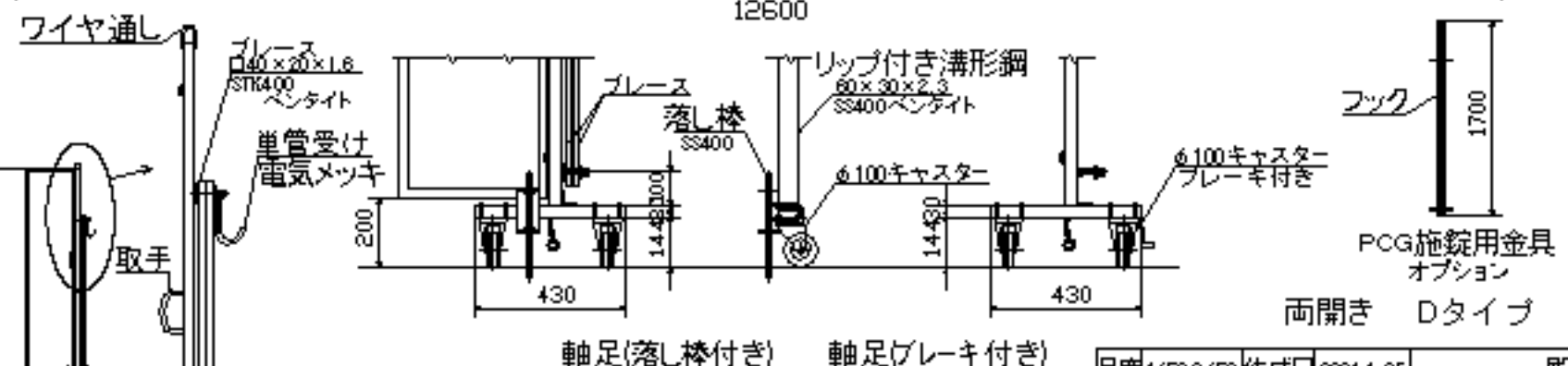
A 矢視
