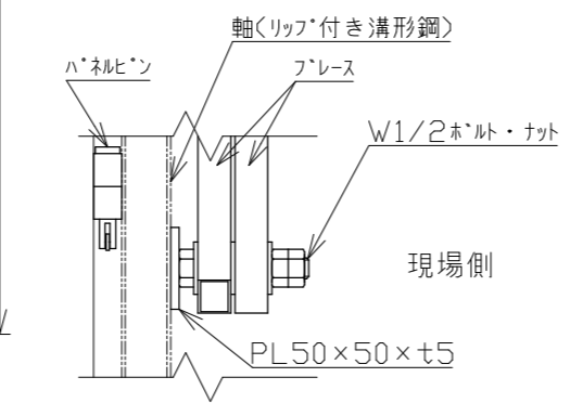
B矢視図 1/5
