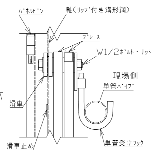
A矢視図 1/5
