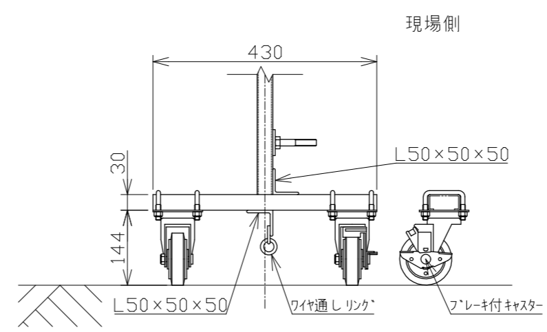
軸足(フレス付き) 1/10
