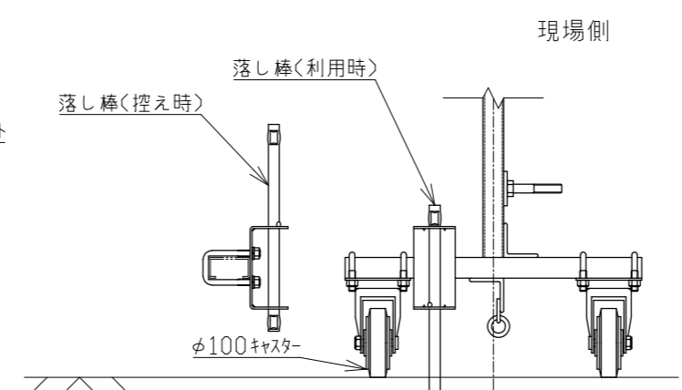
落下棒(オプション) 1/10
