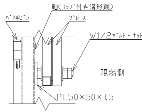
B矢視図 1/5
