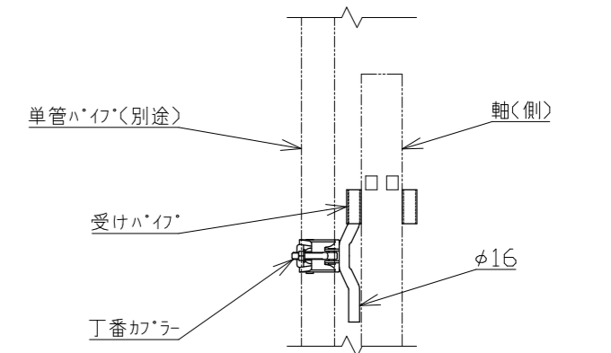
丁番カバー部分詳細 1/10
