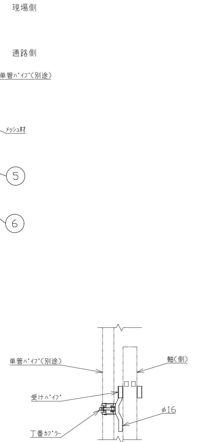
丁番カブラ部分詳細 1/10
